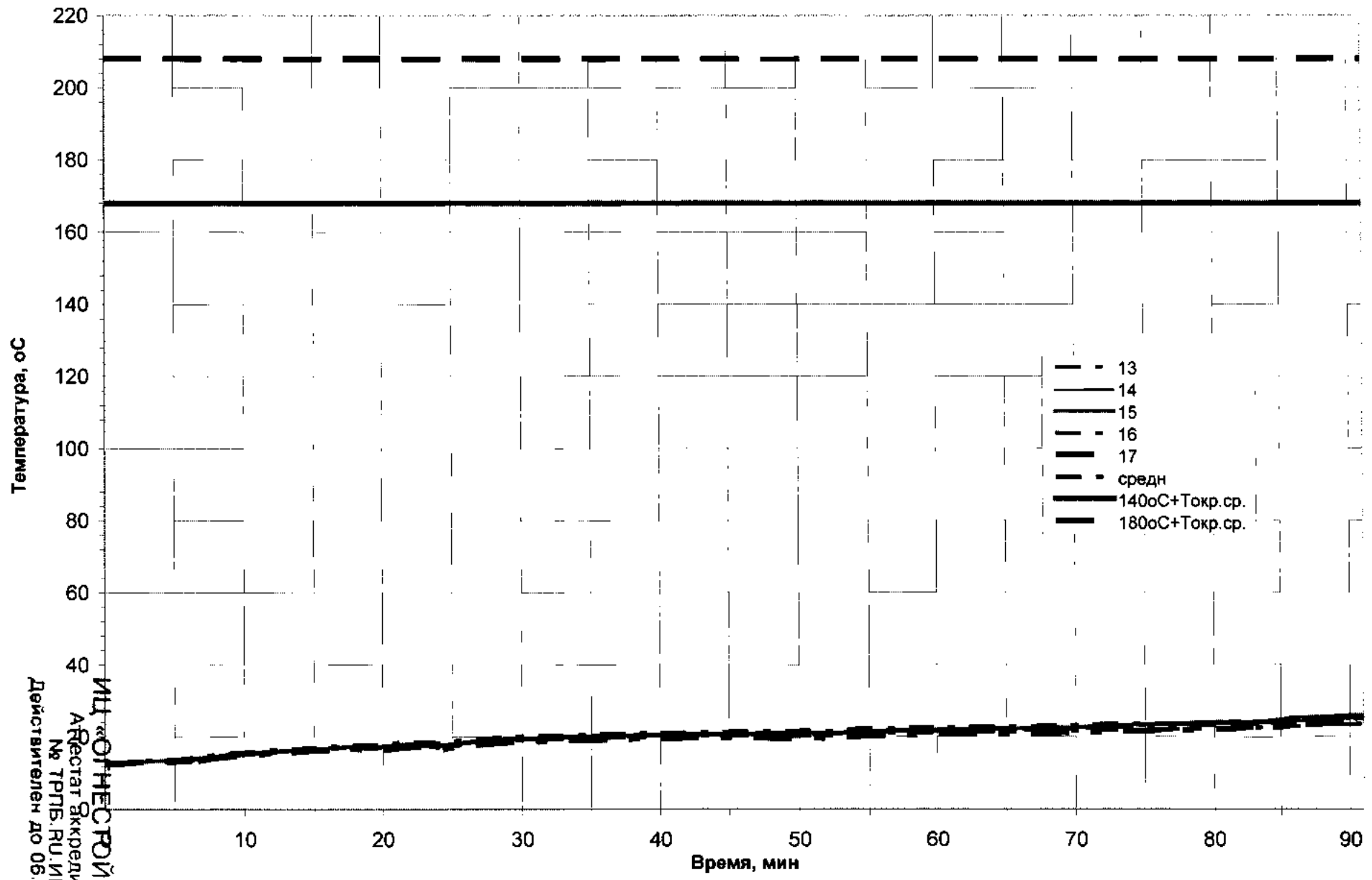
Рис.11. Изменение температуры на необогреваемой поверхности образца №2
